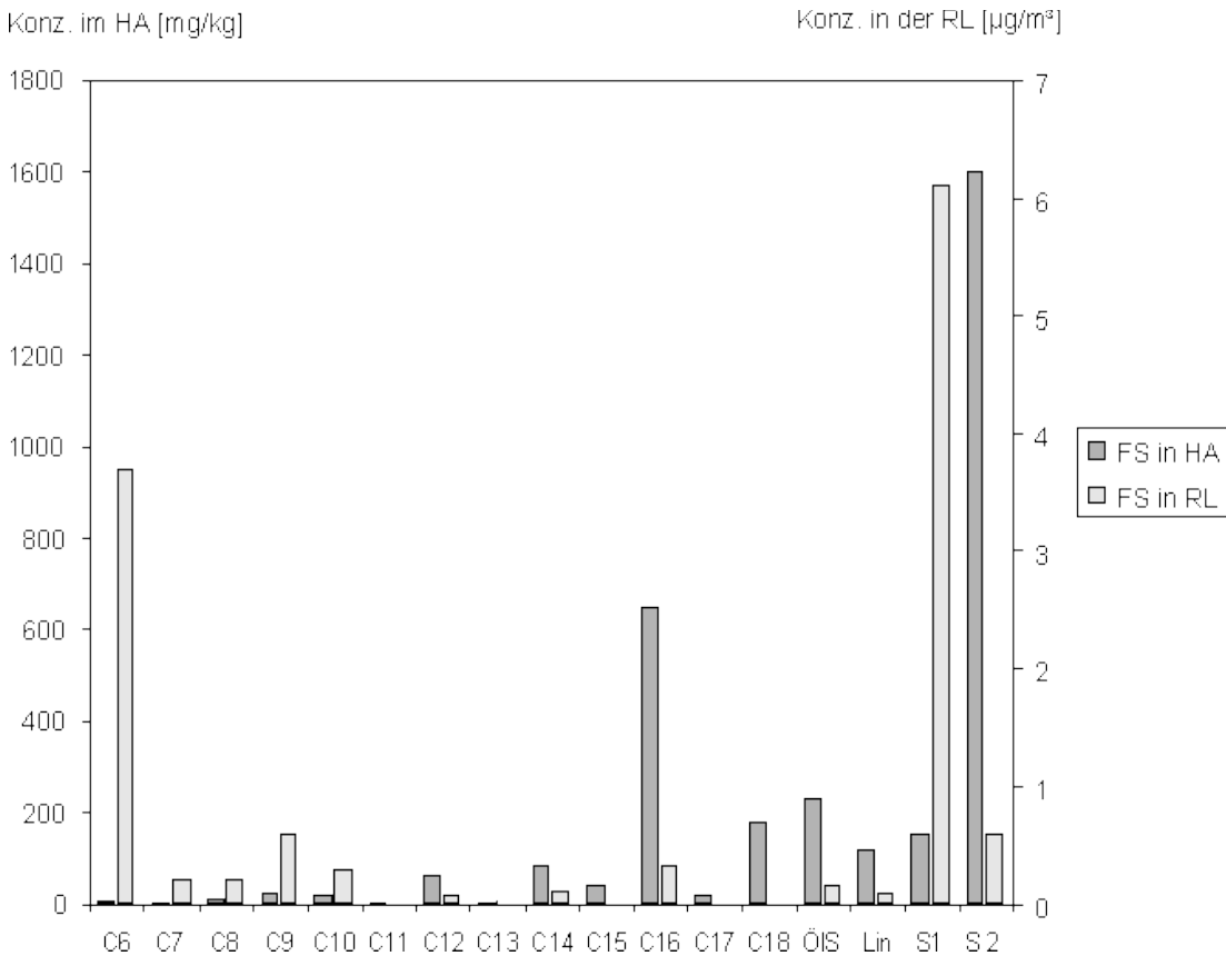
Abbildung 4. Vergleich der Fettsäure-Konzentrationen im Hausstaub und der Raumluft (Median-Werte). Cn - Anzahl der C-Atome der entsprechenden Fettsäure (vgl. Tabelle 1); ÖS - Ölsäure; Lin - Linol/Linolensäure; S1 - Summe C6-C12; S2 - Summe C10 - Linol/en-Säure.
